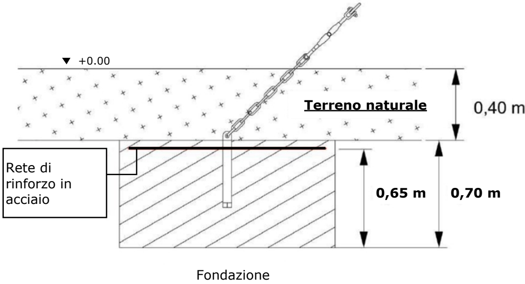
Costruzione della fondazione con rete di rinforzo in acciaio
