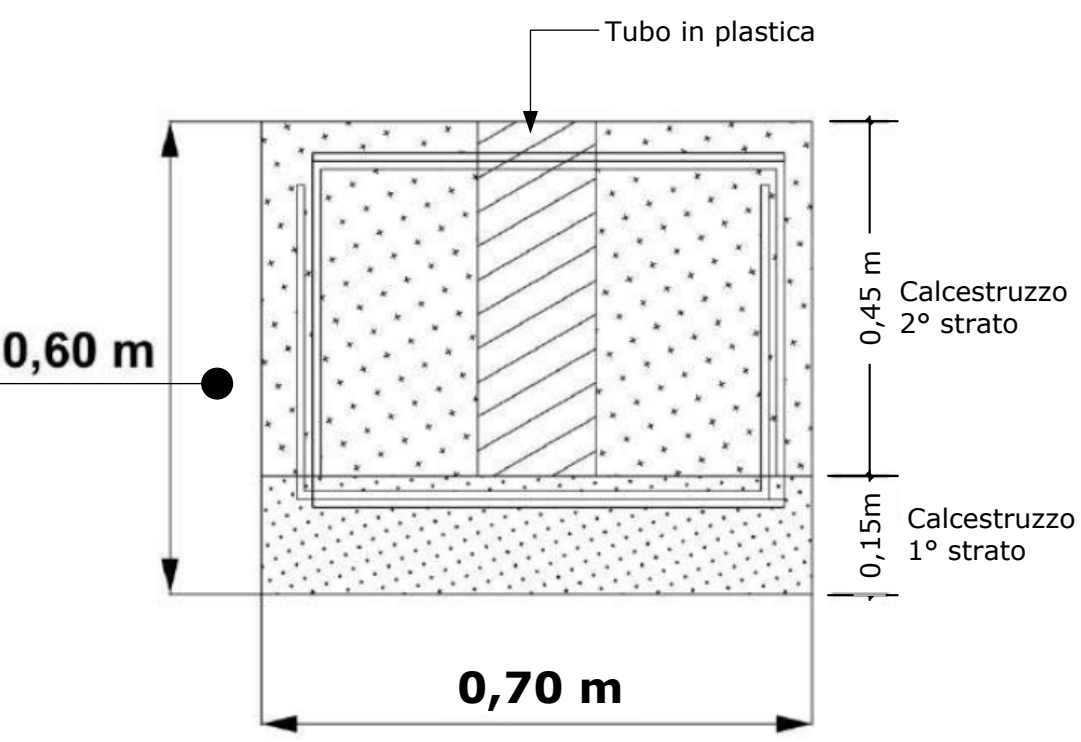
Gabbia di armatura per la fondazione centrale
